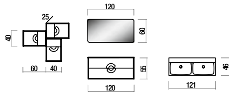
ENCIMERA ARIA DOBLE SENO ARIA COUNTERTOP DOBLE BOWL / PLAN VASQUE ARIA DOUBLE VASQUE
