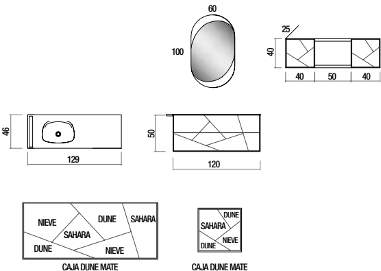
ENCIMERA ORNELLA SENO DESPLAZADO ORNELLA COUNTERTOP BOWL DISPLACED PLAN VASQUE ORNELLA VASQUE DÉPLACÉ
