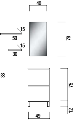
CAJÓN CON DISTRIBUIDOR INTERIOR DRAWER WITH INTERIOR DISTRIBUTOR TIROIR AVEC DISTRIBUTEUR INTÉRIEUR
