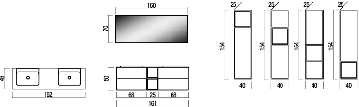
ENCIMERA LOFT DOBLE SENO LOFT COUNTERTOP DOUBLE BOWL PLAN VASQUE LOFT DOBLE VASQUE
