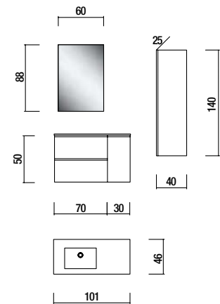
ENCIMERA TIFF SENO DESPLAZADO A LA IZQUIERDA TIFF COUNTERTOP BOWL DISPLACED TO THE LEFT PLAN VASQUE TIFF VASQUE DÉPLACÉ À GAUCHE
