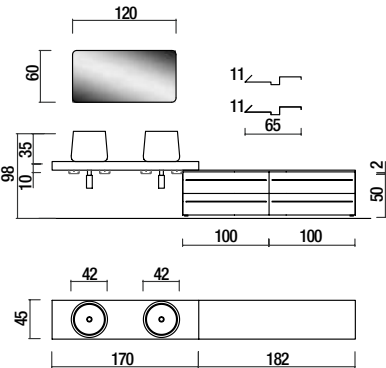
LAVABO CATINO 42 COLOR BLANCO CATINO 42 WASHBASIN WHITE COLOUR / LAVABO CATINO 42 COULEUR BLANC
